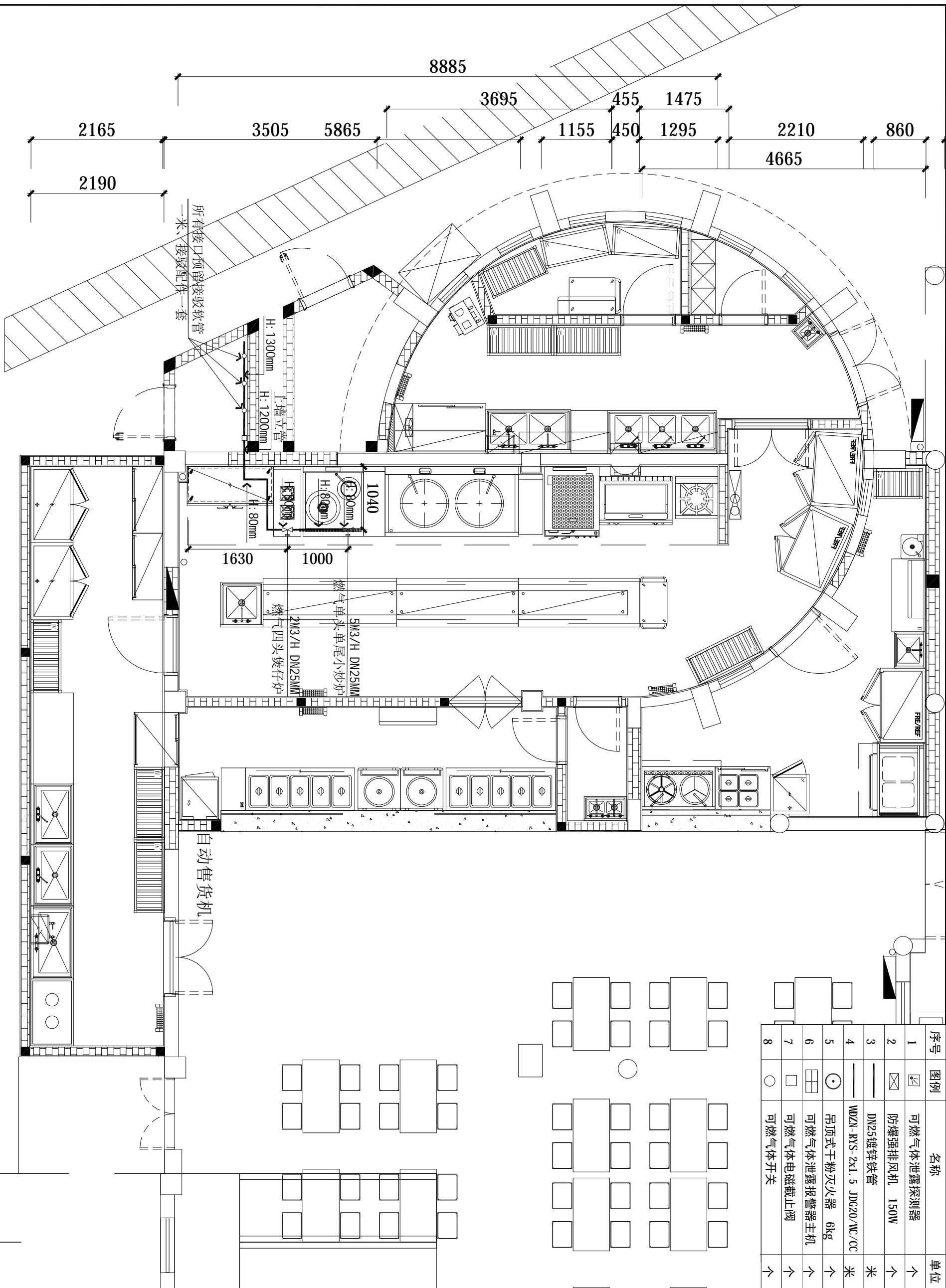
燃气点位布置图 1: 60
