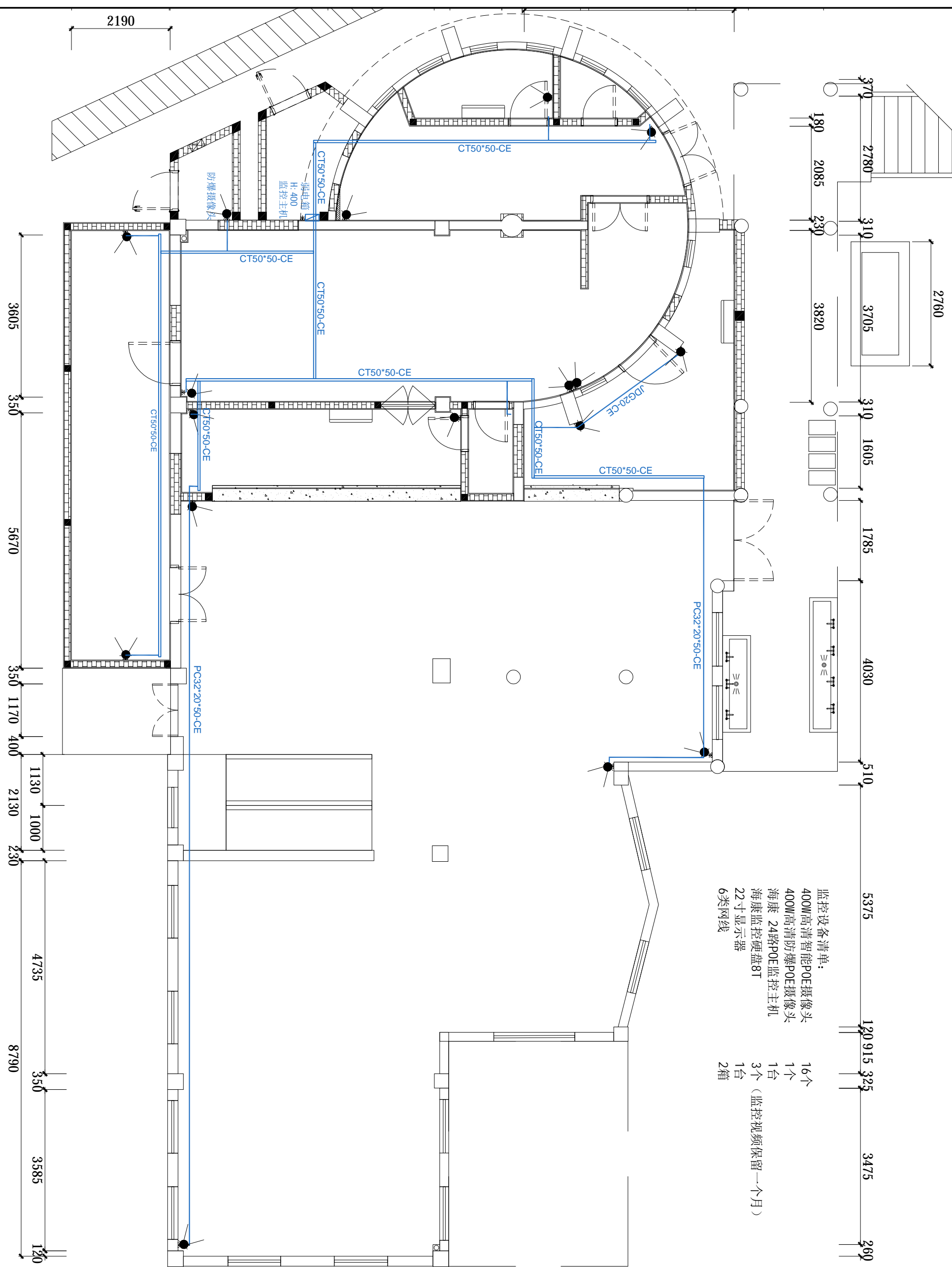
弱电桥架图 1: 80
