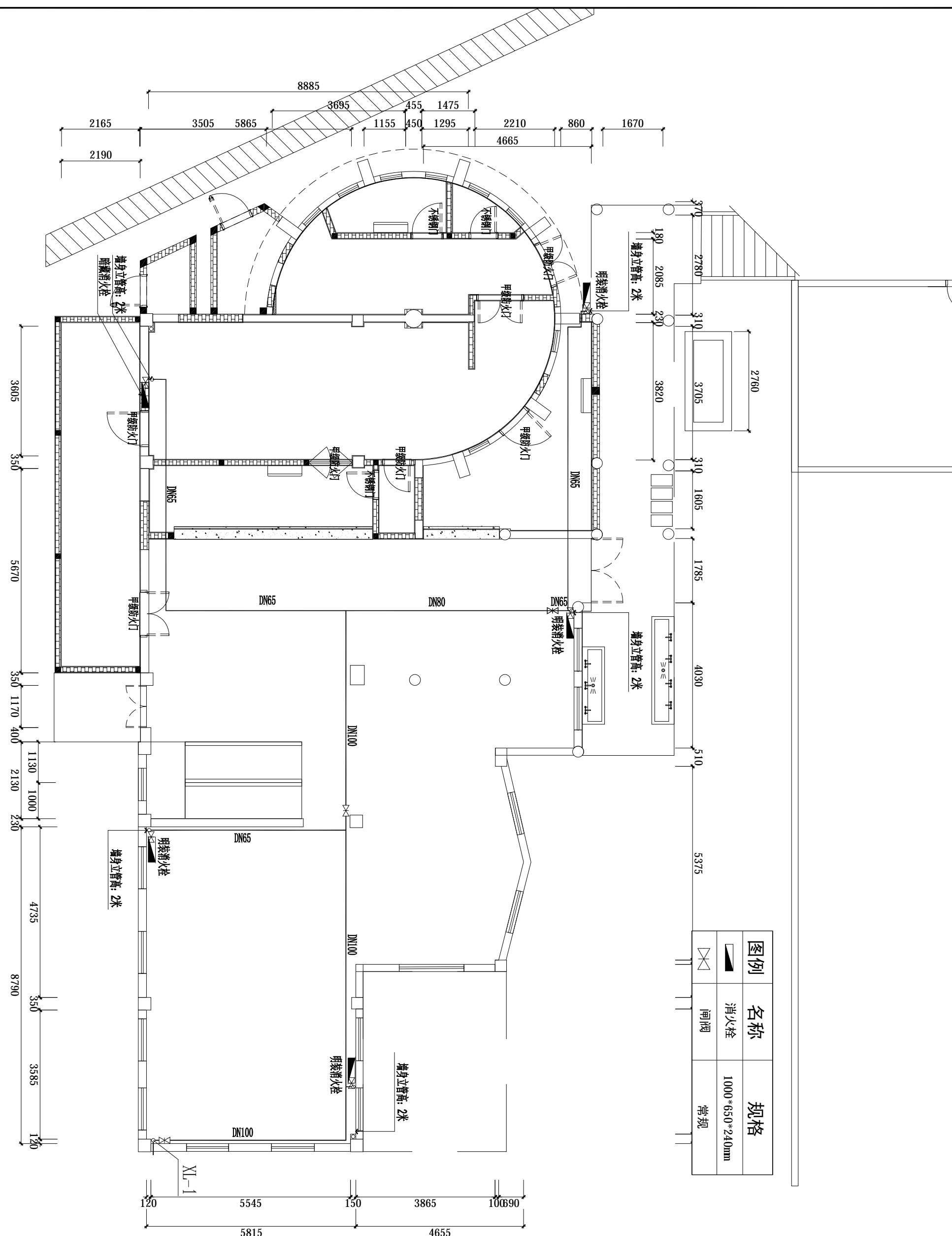
新增消防栓室内走管示意图 1:100
